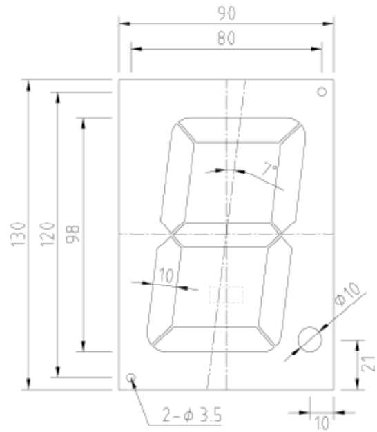
JNR1412A-3 (屋内用)
